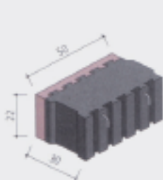
Deckenabschalstein
